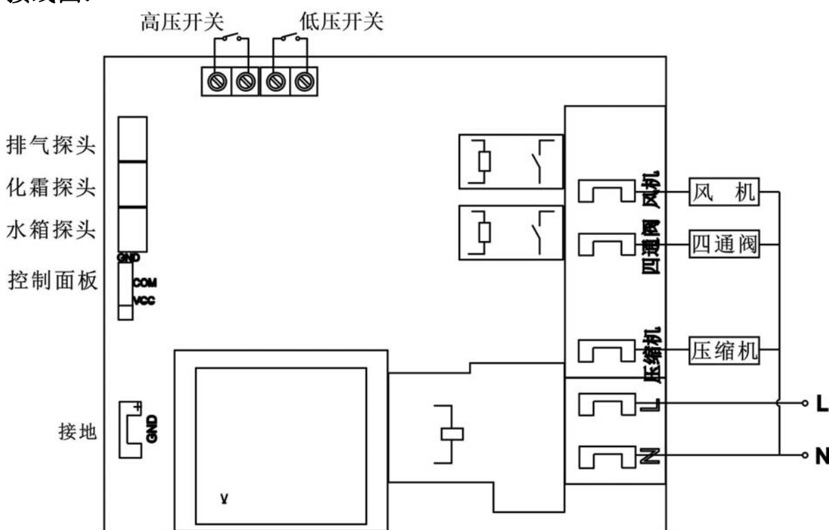
接线图:
