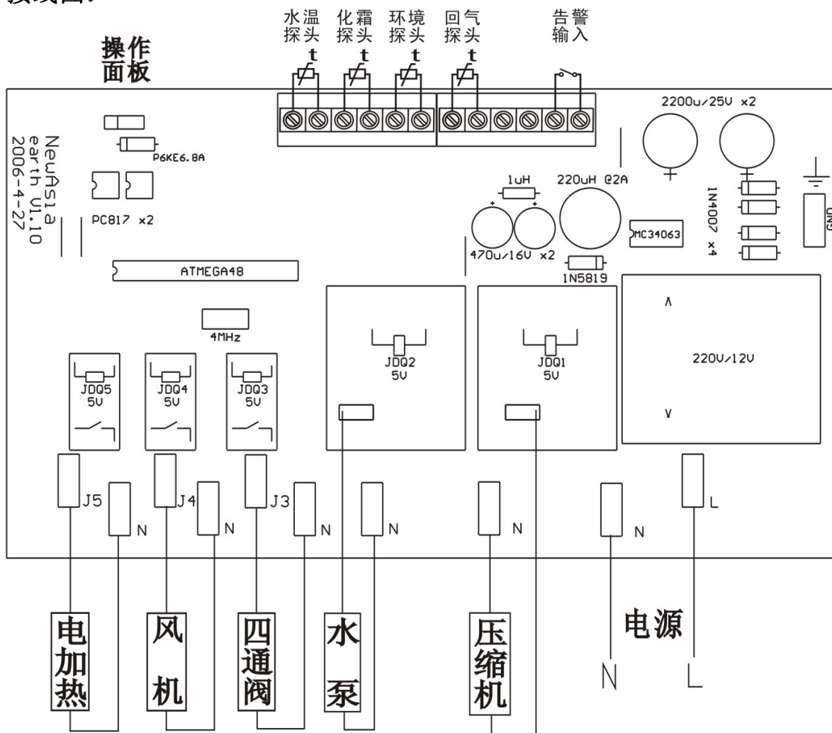
接线图:
